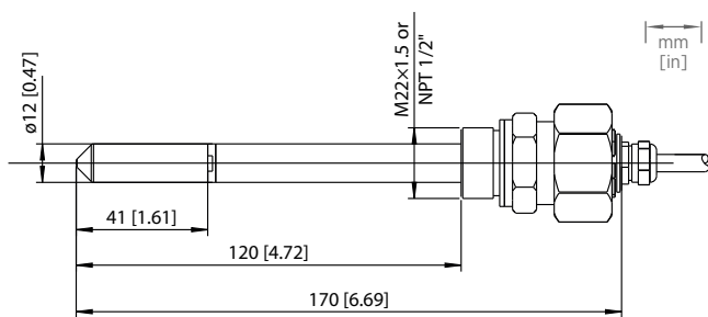
DMP374 dimensions
