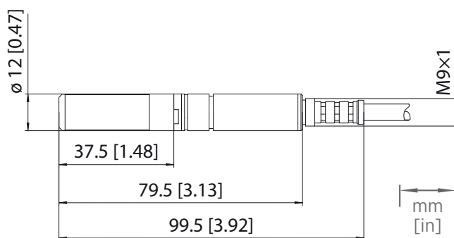
DMP377 dimensions
