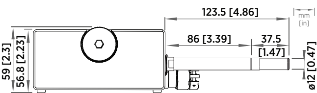
DMP371 dimensions
